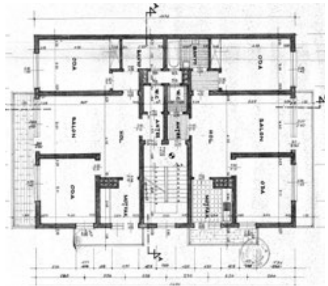
Resim 5: Çatı Katı Planı
